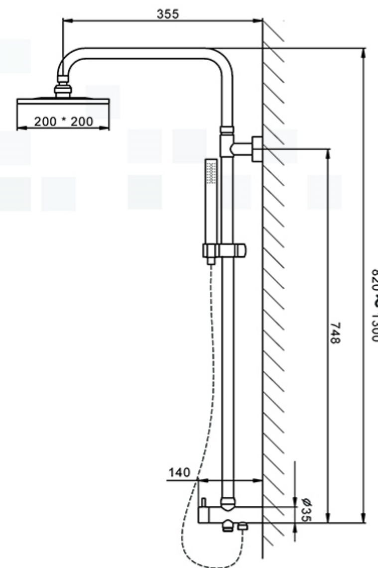
علم یونیک استیل ساخته شده از ( Stainless steel 304 ) کلیه متعلقات شامل : شاور بارانی ، شاور دستی ، براکت ، هلدرو شیلنگ از جنس استیل 304 می باشند. Code : 6356-BR-80S1
