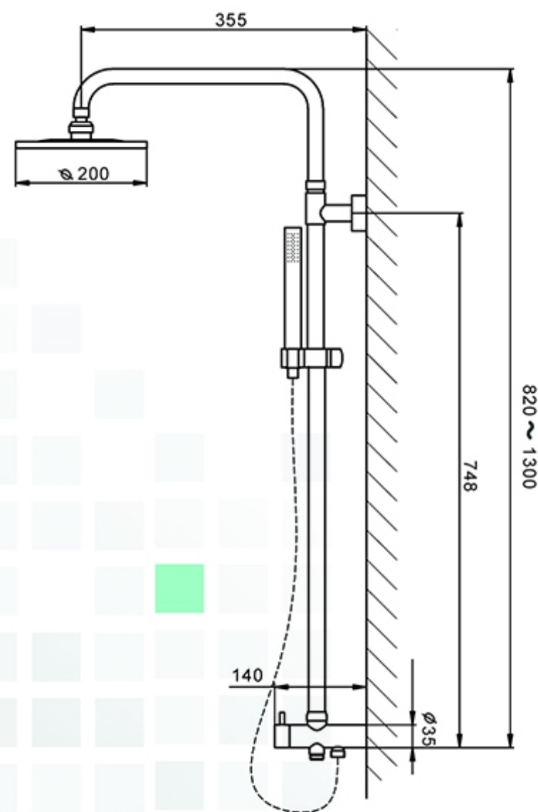
علم یونیک استیل ساخته شده از ( Stainless steel 304 ) کلیه متعلقات شامل : شاور بارانی ، شاور دستی ، براکت ، هلدرو شیلنگ از جنس استیل 304 می باشند. Code : 6355-BR-80S1
