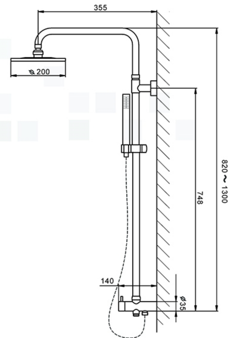
علم یونیک کروم دارای سیستم تنظیم ارتفاع علم ساخته شده از برنج با روکش کروم Code : 6349-BR-82CP
